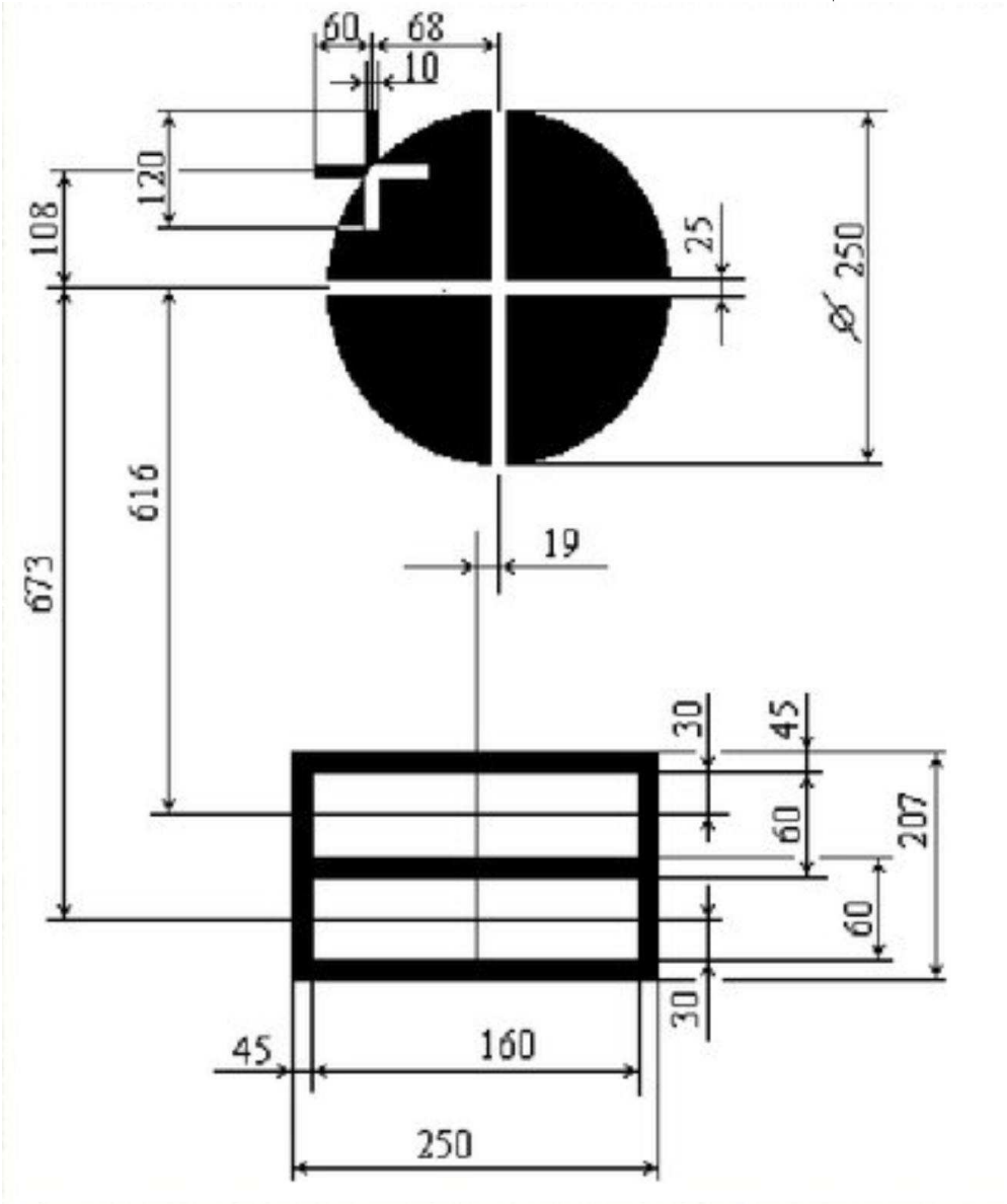
СХЕМА ВЫВЕРОЧНОЙ МИШЕНИ ДЛЯ ПРОВЕРКИ ОПТИЧЕСКОГО И МЕХАНИЧЕСКОГО ПРИЦЕЛОВ
