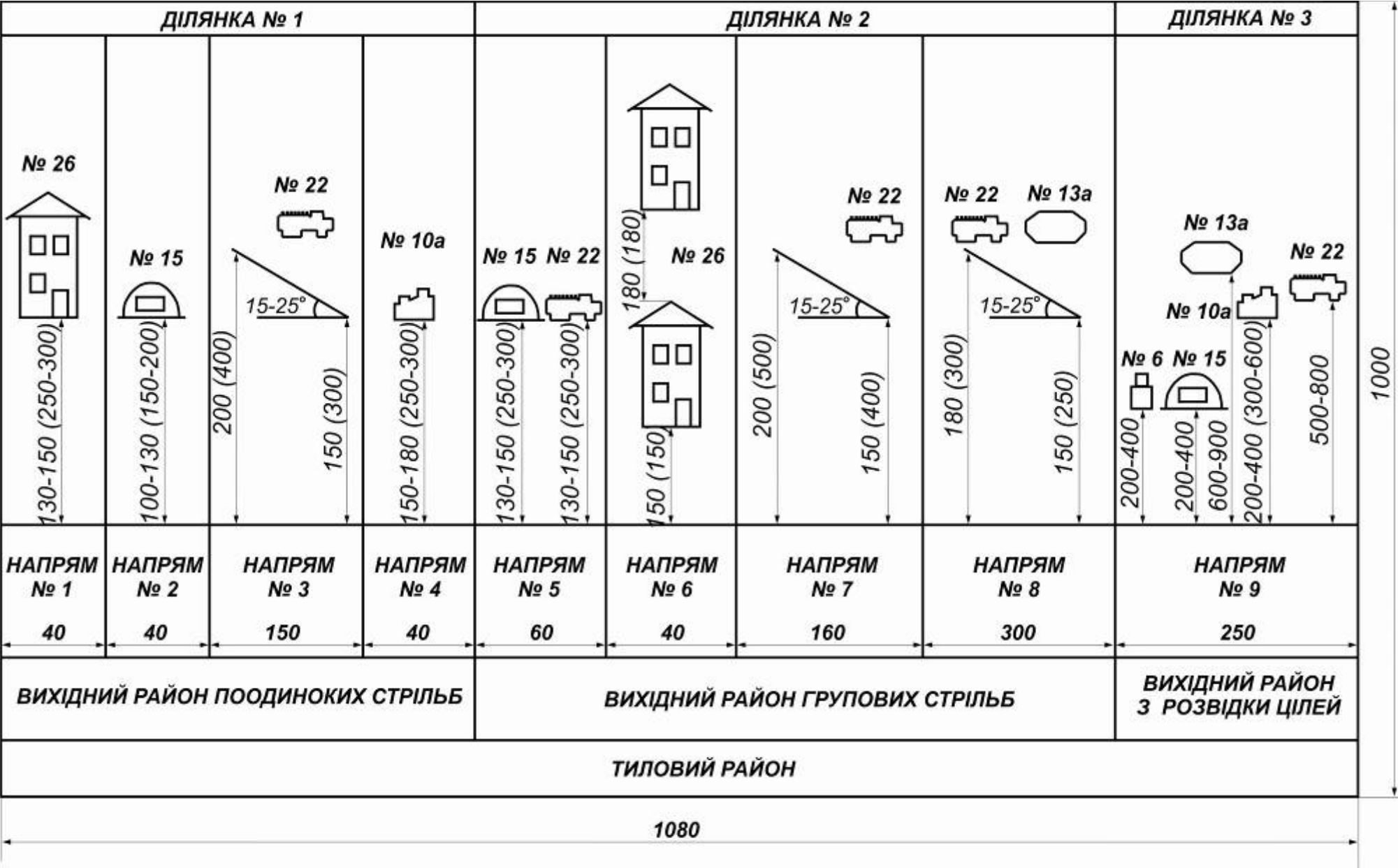
Рисунок Д13.1 – Варіант обладнання полігону для стрільби з вогнеметів.
