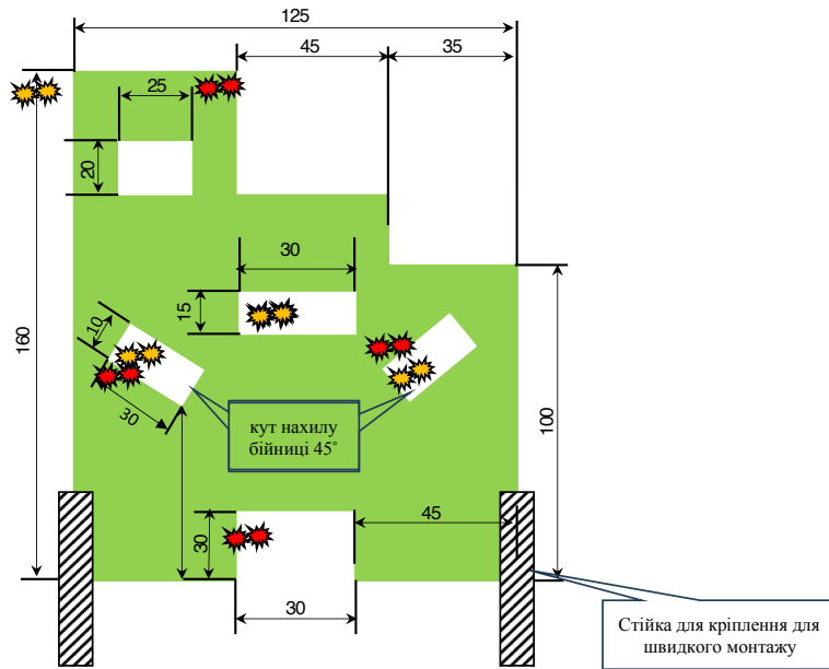
СХЕМА ОБЛАДНАННЯ УКРИТТЯ
