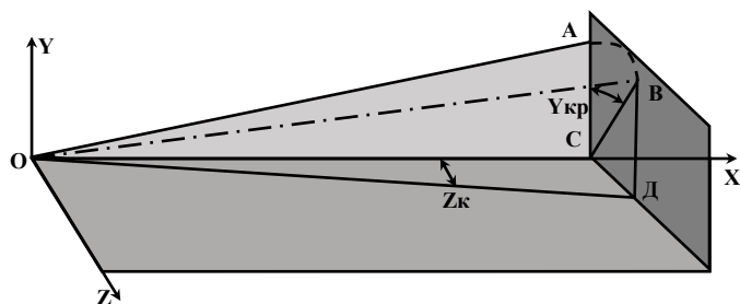
Рисунок 14 – вплив бічного крену БМ політ снаряда.
