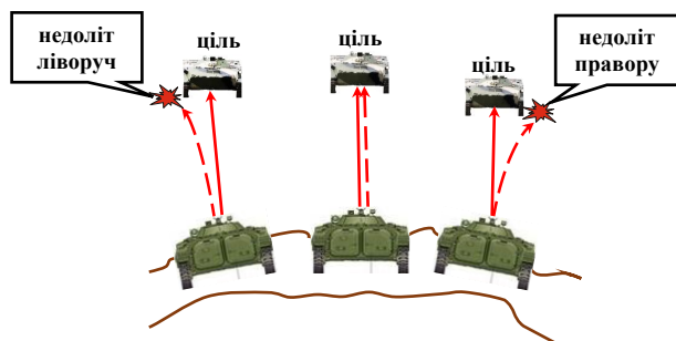
Рисунок 14 – вплив бічного крену БМ політ снаряда.
