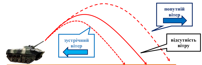
Рисунок 13 – вплив зустрічного (попутного) вітру на дальність польоту снаряда.
