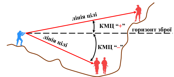
Рисунок 16 – вплив кута місця цілі (КМЦ).
