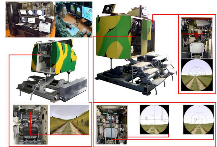
Рисунок 19 – комплексний тренажер екіпажу БМП-2.
