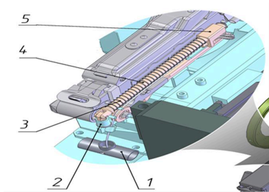
Рисунок 6.8.9.2 – механізм ручного заряджання кулемета.
